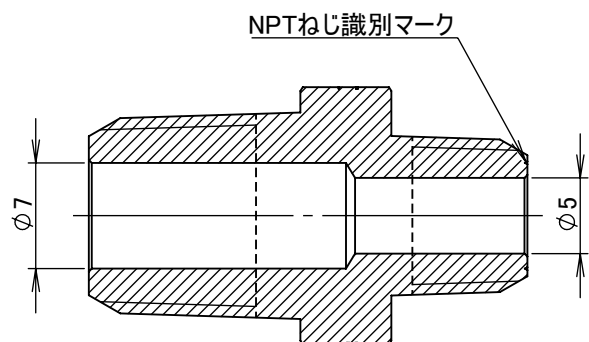
断面図 A-A
