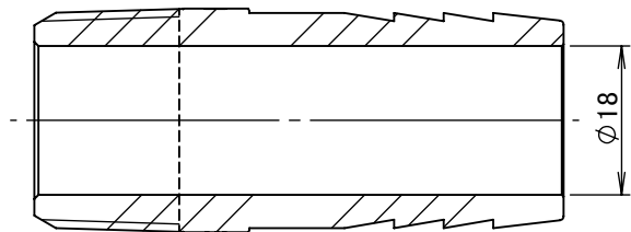
断面図 A-A
