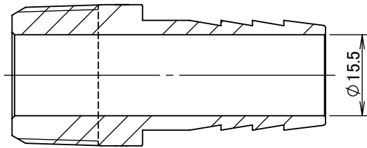
断面図 A-A
