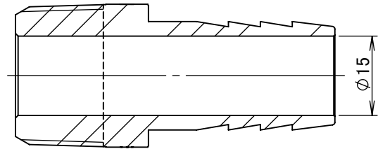
断面図 A-A
