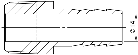
断面図 A-A
