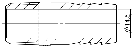
断面図 A-A
