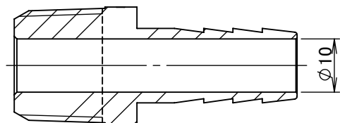
断面図 A-A
