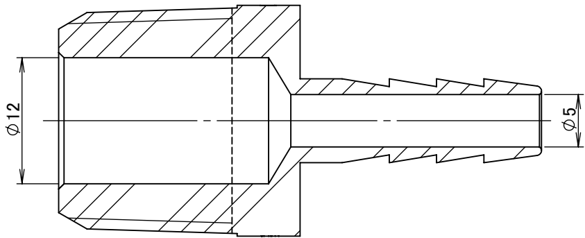
断面図 A-A
