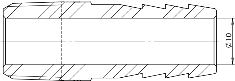
断面図 A-A
