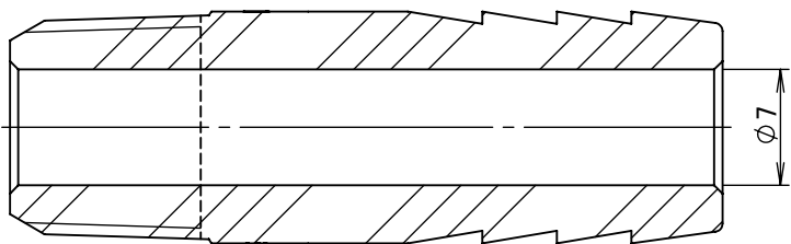
断面図 A-A
