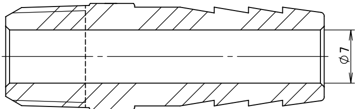
断面図 A-A
