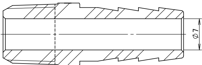
断面図 A-A
