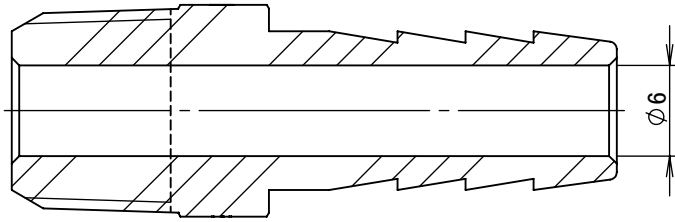
断面図 A-A
