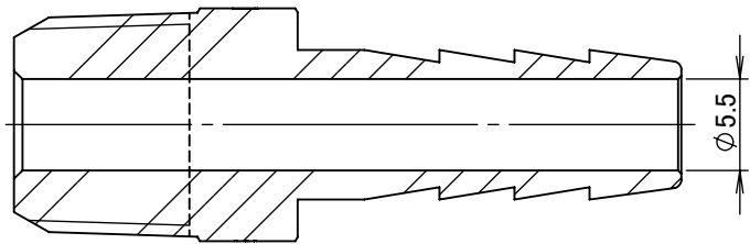
断面図 A-A
