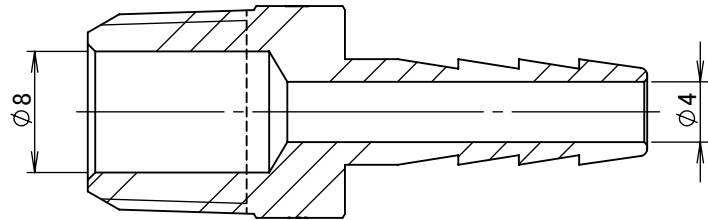
断面図 A-A
