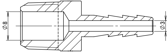
断面図 A-A
