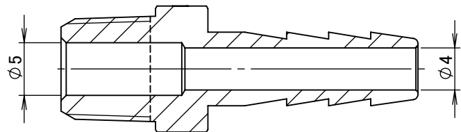
断面図 A-A
