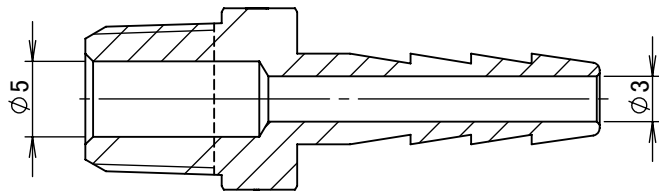
断面図 A-A
