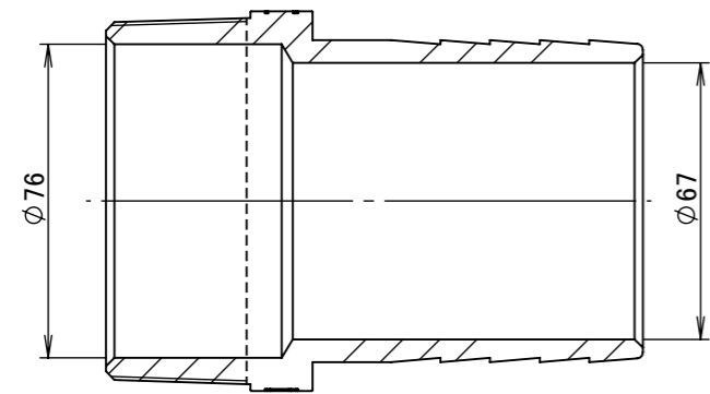
断面図 A-A
