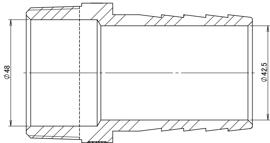
断面図 A-A
