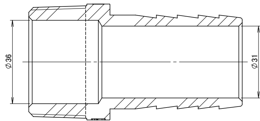
断面図 A-A
