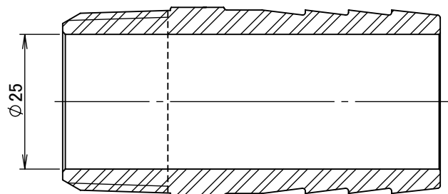
断面図 A-A
