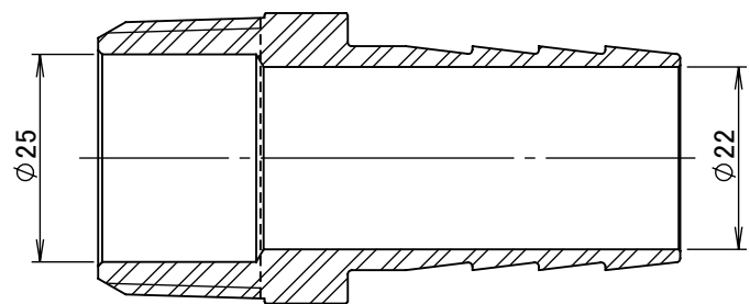
断面図 A-A
