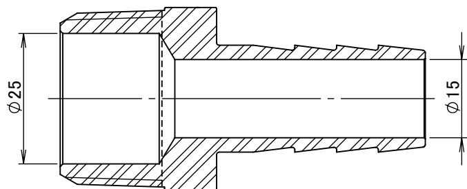
断面図 A-A
