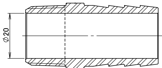
断面図 A-A
