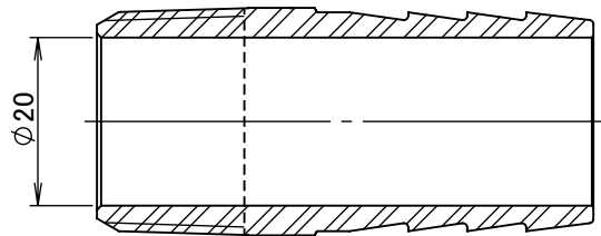
断面図 A-A
