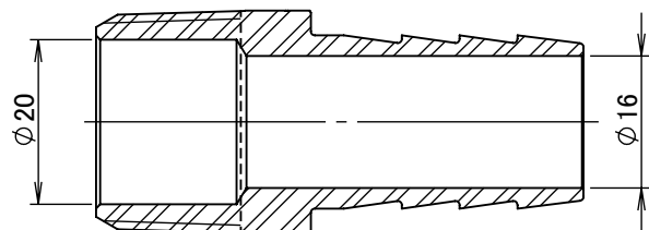
断面図 A-A
