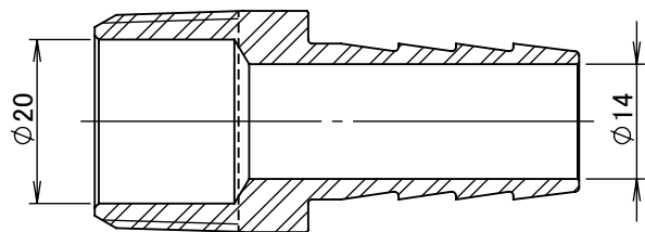
断面図 A-A
