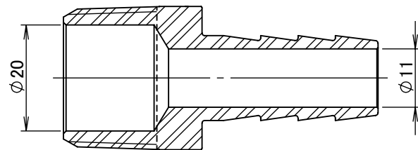
断面図 A-A
