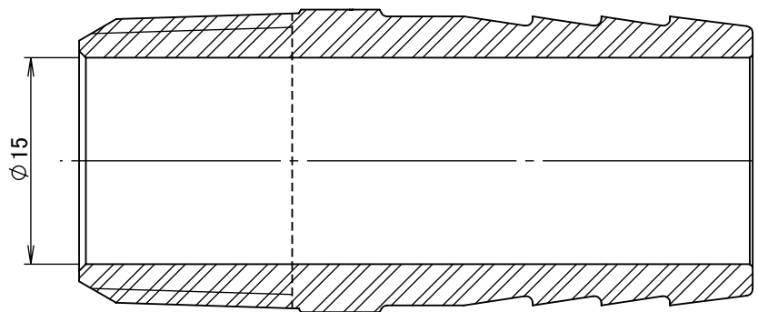
断面図 A-A
