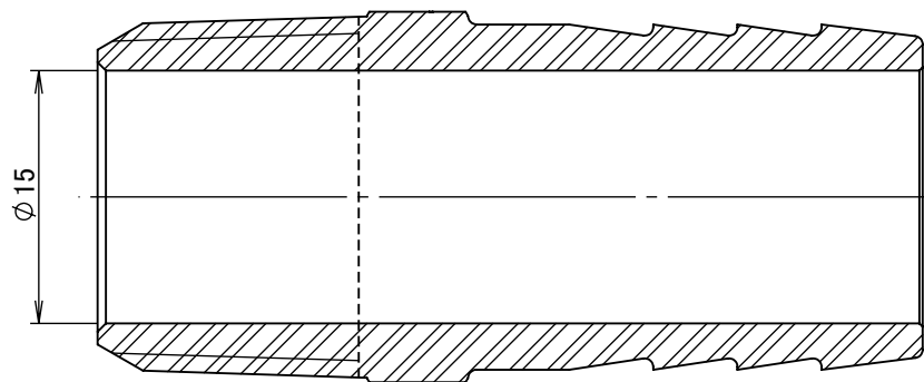
断面図 A-A
