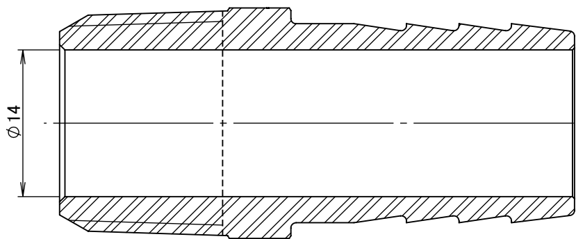
断面図 A-A
