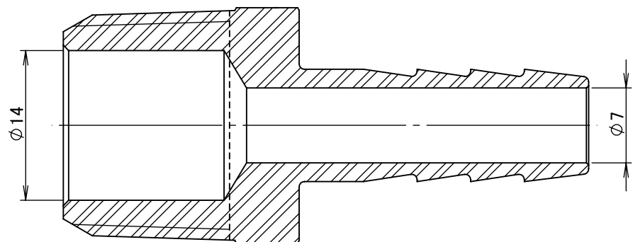
断面図 A-A
