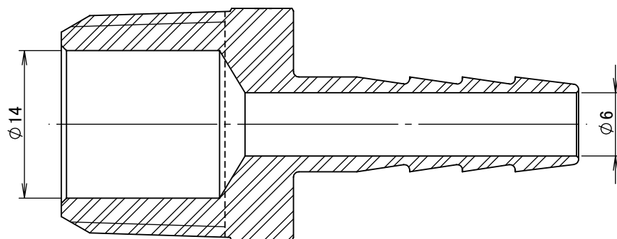
断面図 A-A
