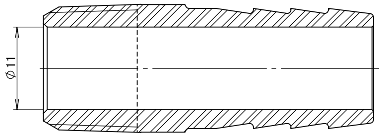
断面図 A-A
