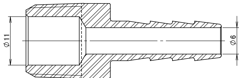
断面図 A-A
