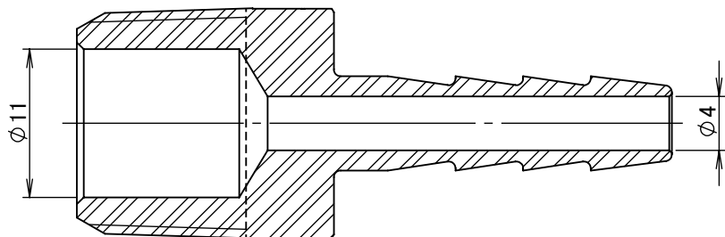
断面図 A-A
