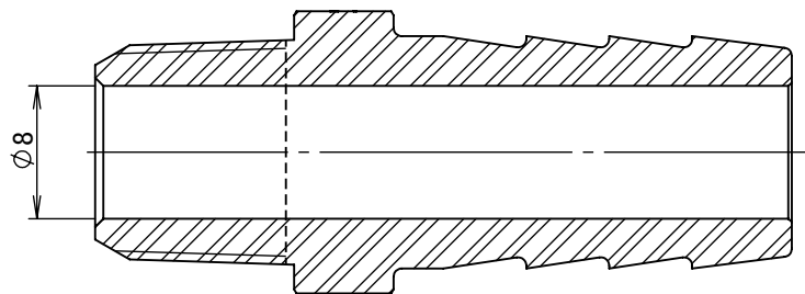
断面図 A-A
