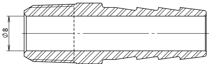
断面図 A-A
