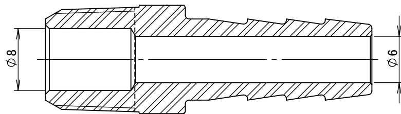
断面図 A-A
