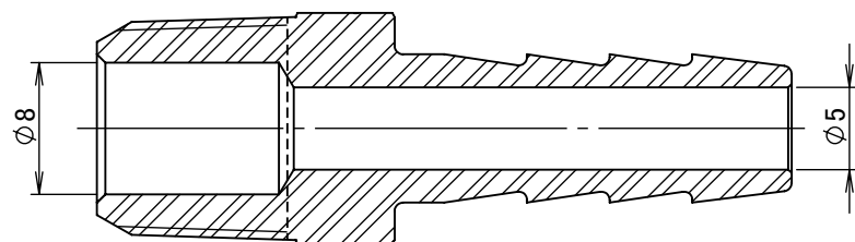
断面図 A-A
