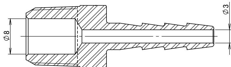
断面図 A-A
