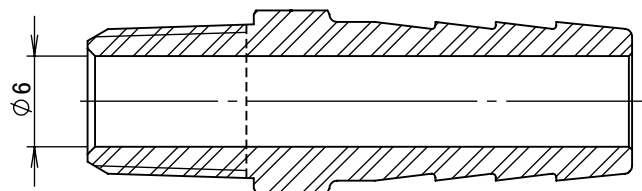
断面図 A-A
