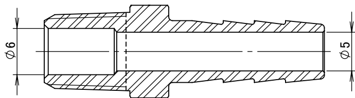
断面図 A-A
