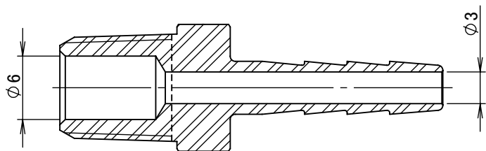
断面図 A-A
