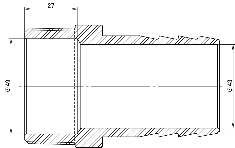
断面図 A-A
