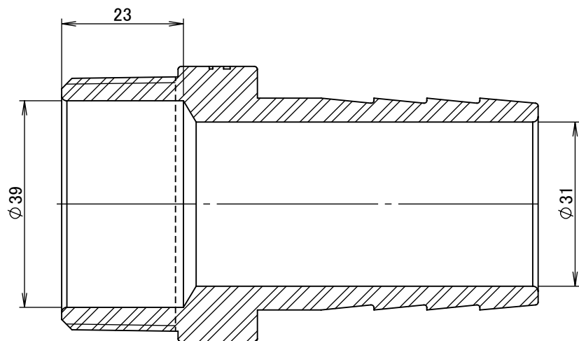
断面図 A-A
