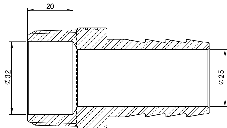
断面図 A-A
