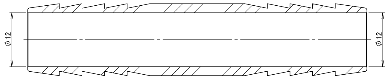
断面図 A-A
