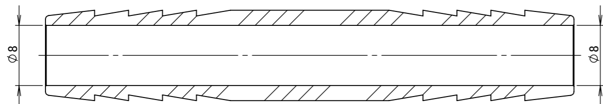
断面図 A-A
